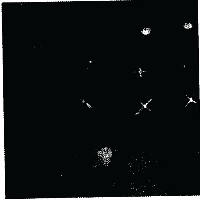
الشكل (84): ضوء يمر خلال بلورة من الكالسايت (حجر آيسلاندا) يأخذ ممرات مختلفة وفق حالة استقطابه وتوضع البلورة.
